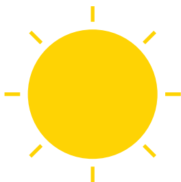
le Soleil
