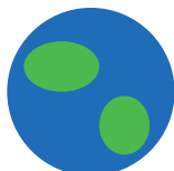
la Terre
